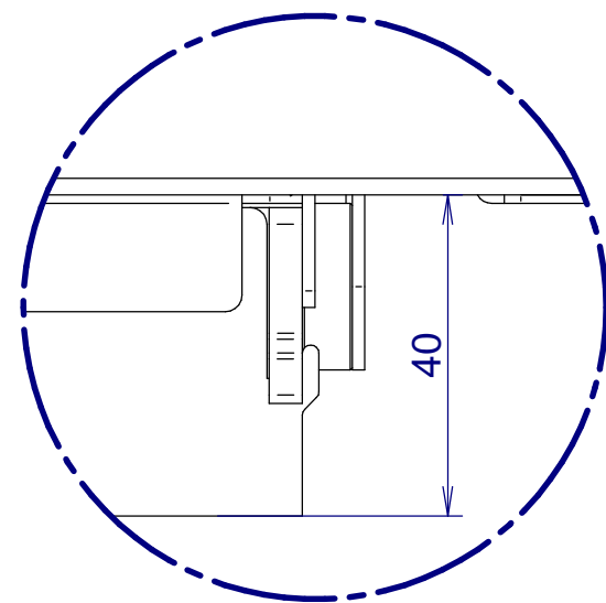
DETAIL A 1:1
